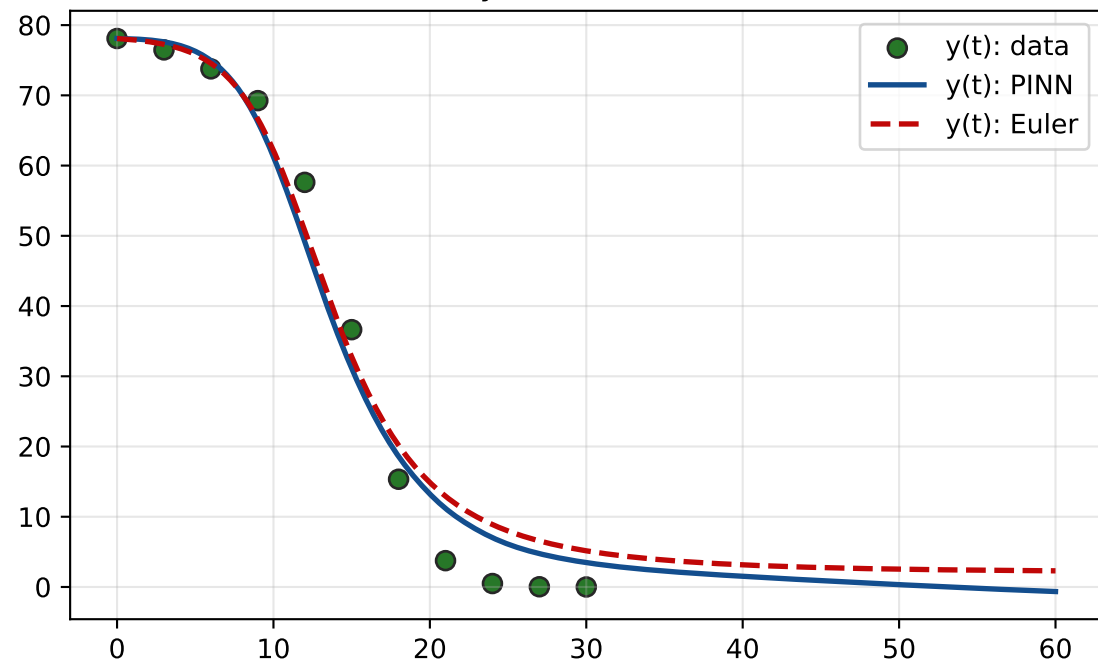
y(t): Fructose
